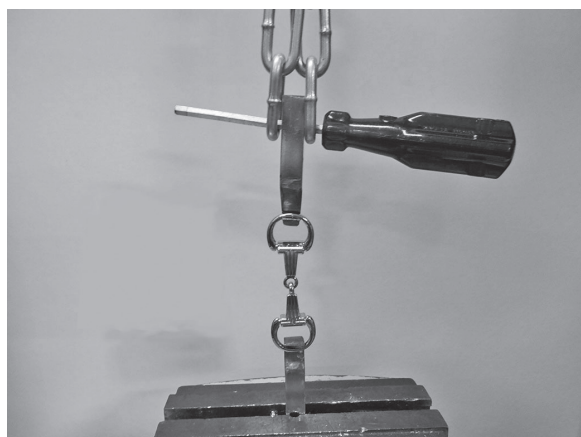
図3 引張強さ試験（美錠）
